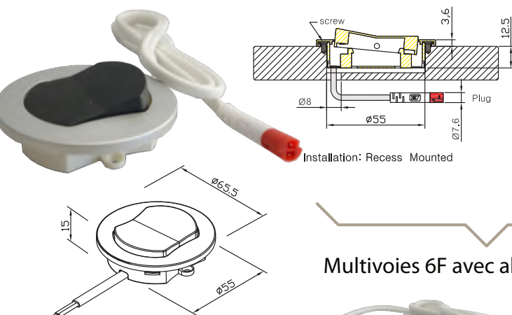
33258 Kit interrupteur à encastrer
