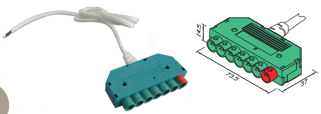
Multivoies 6F avec alimentation
